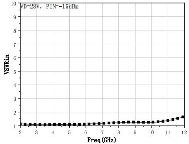
VSWRin
