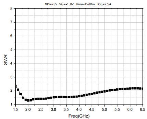
VSWRin
