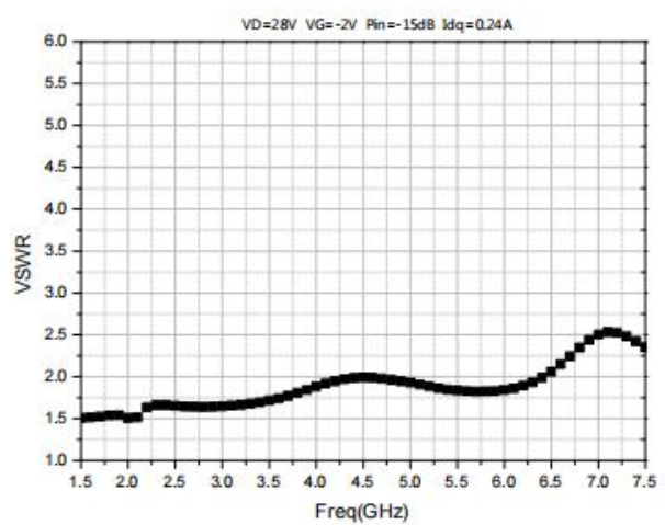
VSWRin
