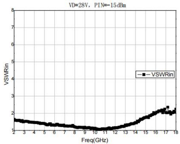
VSWRin
