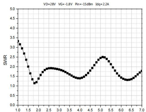
VSWRin
