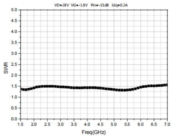
VSWRin
