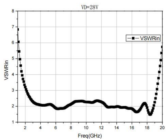
VSWRin
