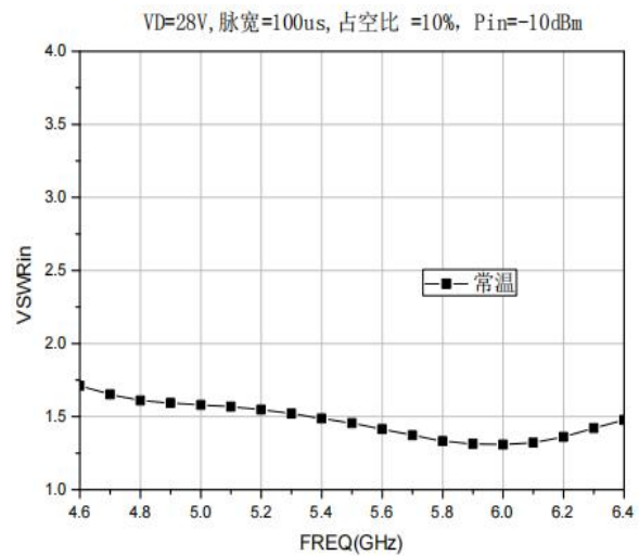
VSWRin
