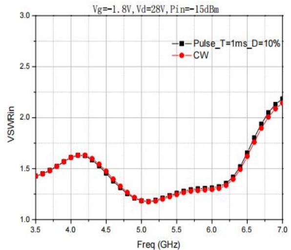
VSWRin
