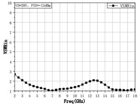
VSWRin
