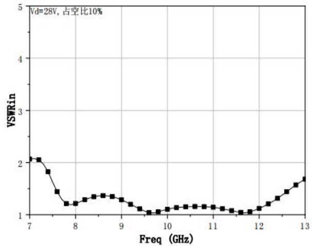
VSWRin
