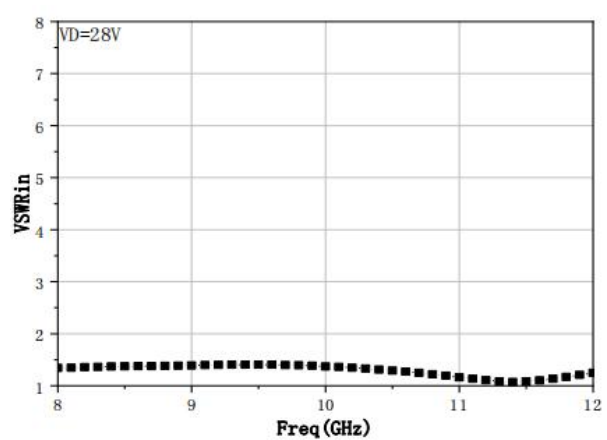
VSWRin
