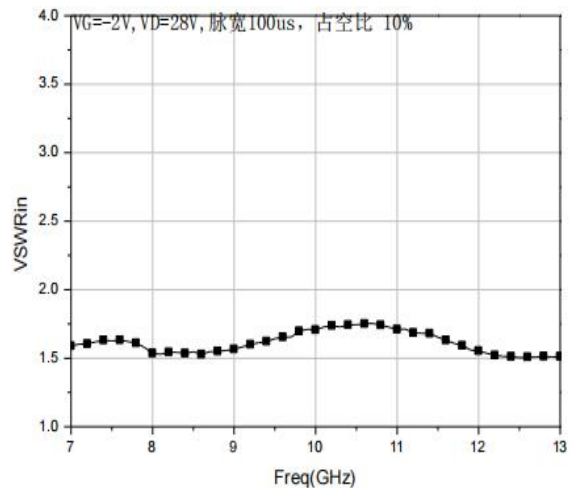
VSWRin
