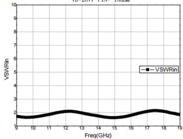
VSWRin
