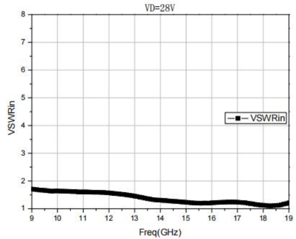
VSWRin
