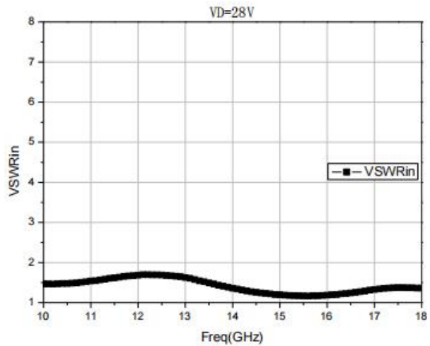
VSWRin
