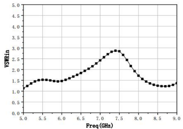
VSWRin
