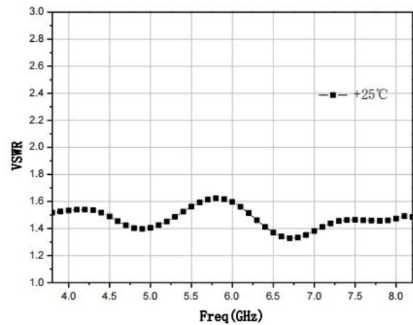
VSWRin
