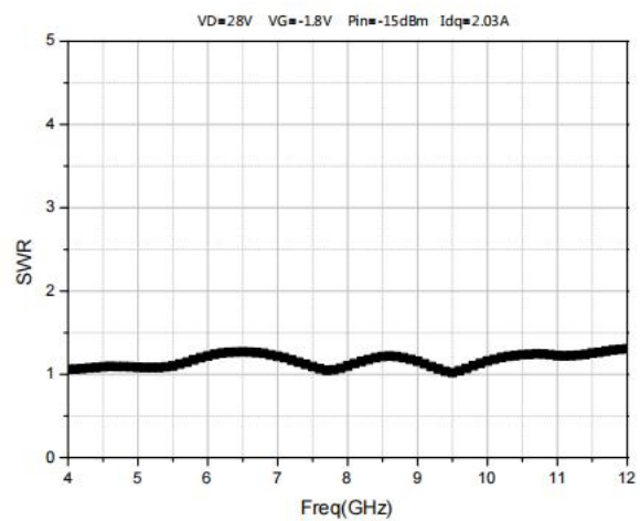
VSWRin
