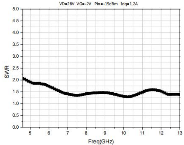
VSWRin
