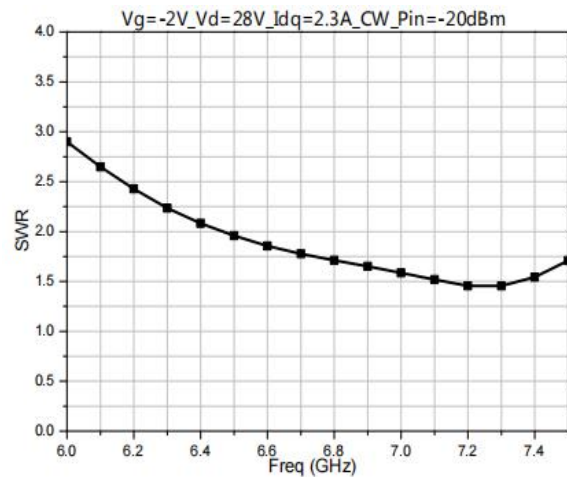
VSWRin
