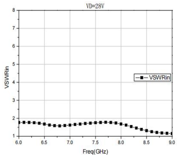
VSWRin
