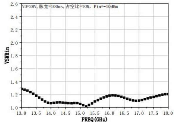
VSWRin
