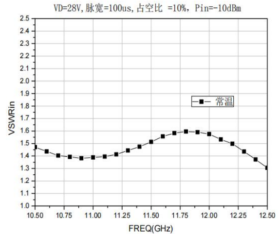
VSWRin
