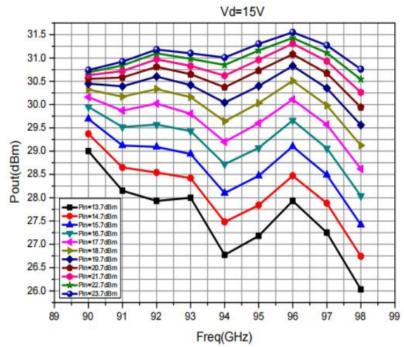
Pout
