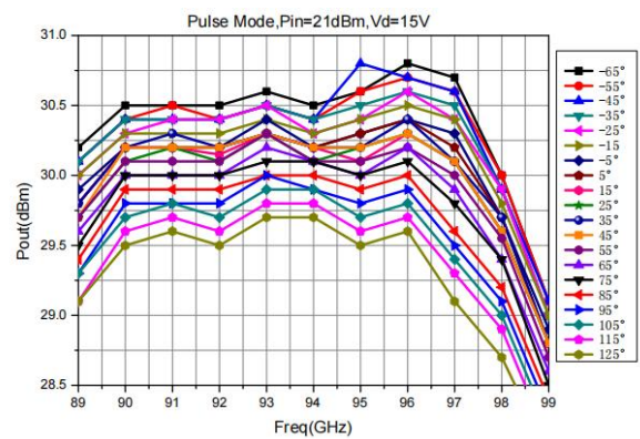
Pout
