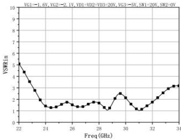
VSWRin
