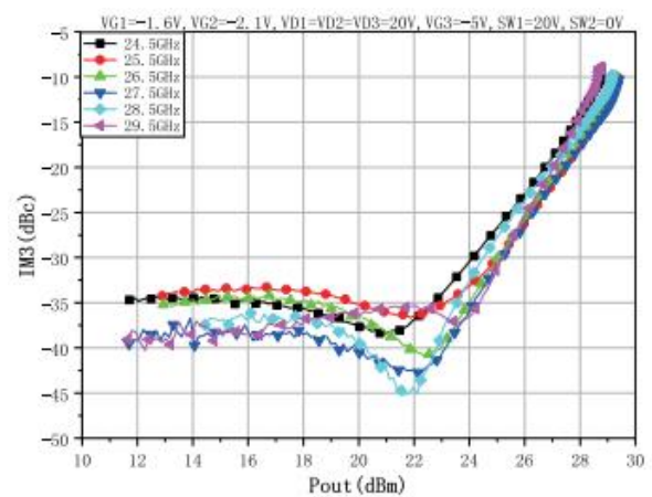
IM3
