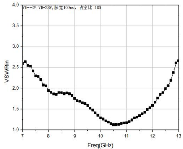
VSWRin
