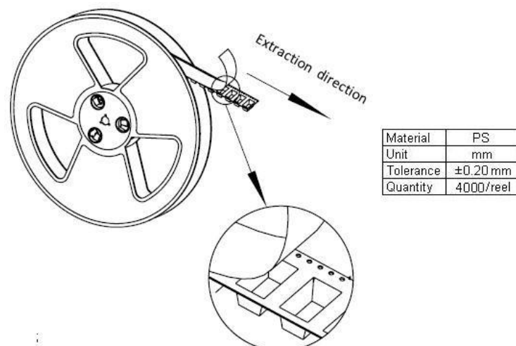
Reel Dimensions
