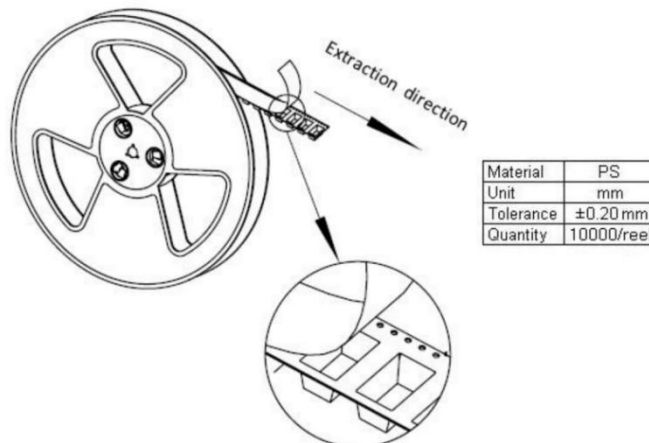
Reel Dimensions
