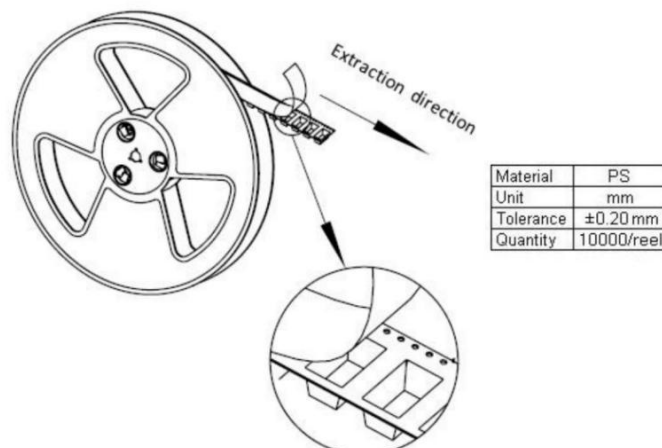
Reel Dimensions
