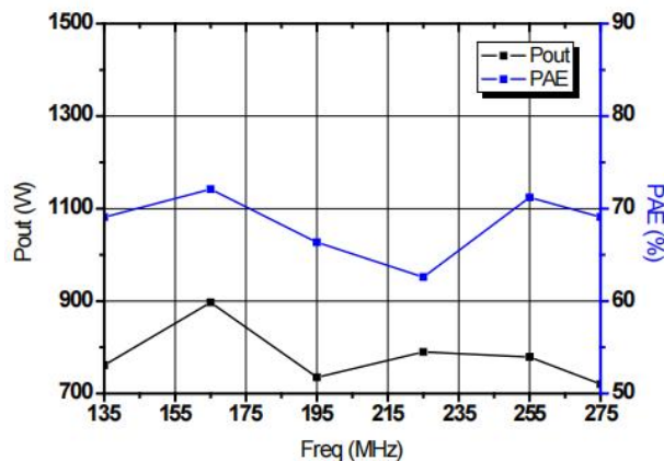
Pout、PAE&Freq.
