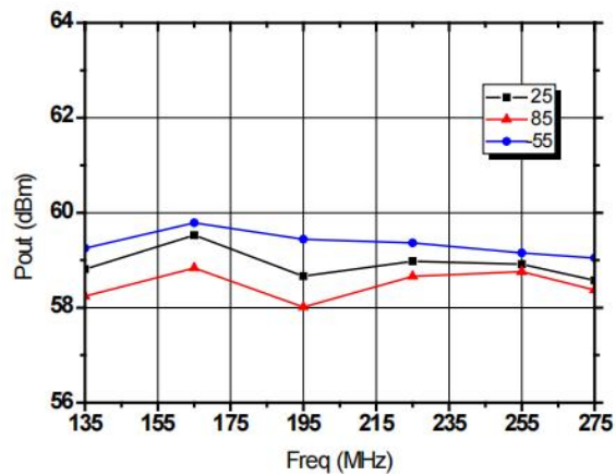
Pout、PAE&Freq.
