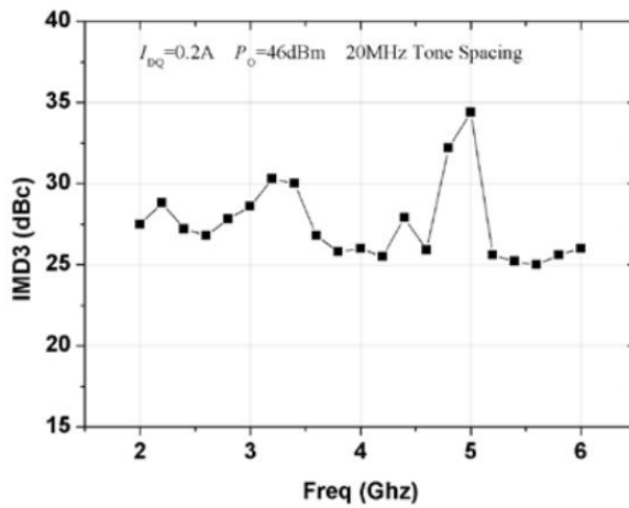
IMD3 40W
