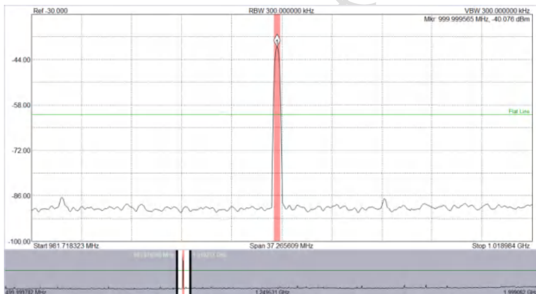
图35：区域缩放用于事件的仔细检查。
