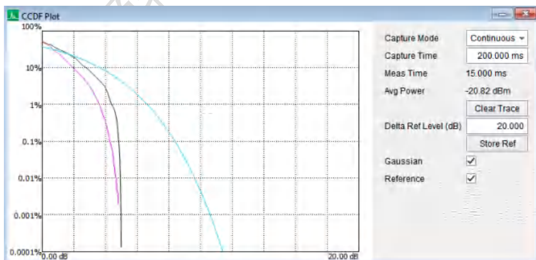
图10：将合成噪声信号与高斯参考信号和理想测试信号进行比较
