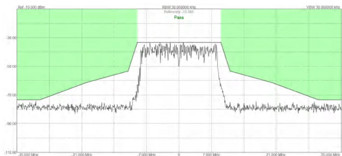
图42：针对802.11 OFDM传输掩码测试输入
